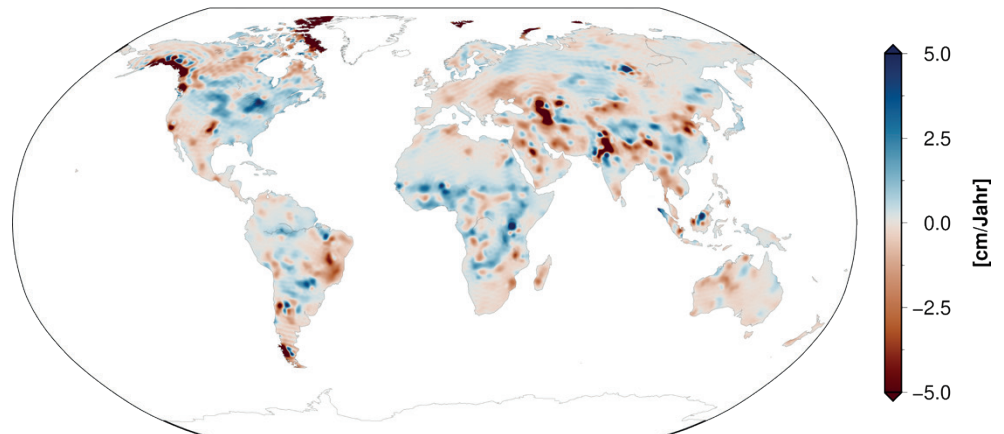
Weltkarte: Trend zur Gesamtwasserspeicherung (2002–2021). In rot sind die Regionen mit Wasserdefizit, in blau mit Wasserüberschuss markiert. (Karte: E. Börgens/GFZ)
